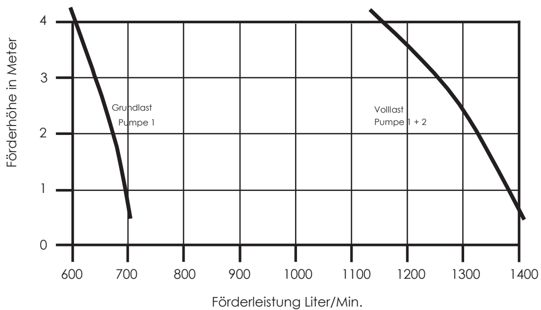
RKS 800 (1200)Leistungsdaten mit SP700 der Doppelpumpanlage Grundlast - Volllast
