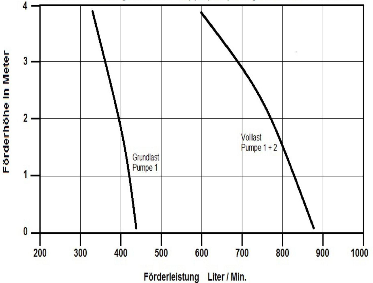
RKS 800 Leistungsdaten der Doppelpumpanlage Grundlast - Volllast
